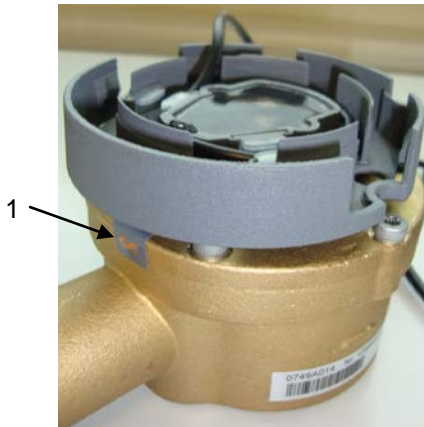
Sigilli di fabbrica sulla volumetrica (1) e la sonda di temperatura (2) del Superstatic 749
