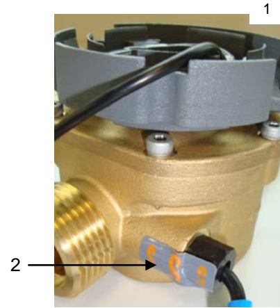
Sigilli di fabbrica sulla volumetrica (1) e la sonda di temperatura (2) del Superstatic 749
